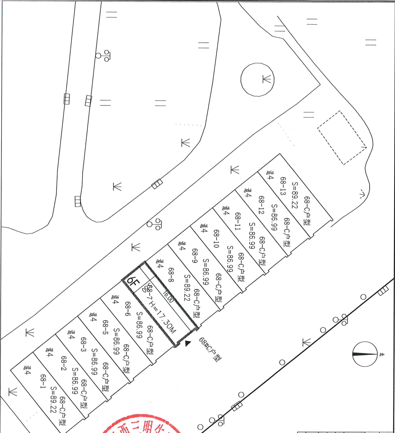
总平面布置图
