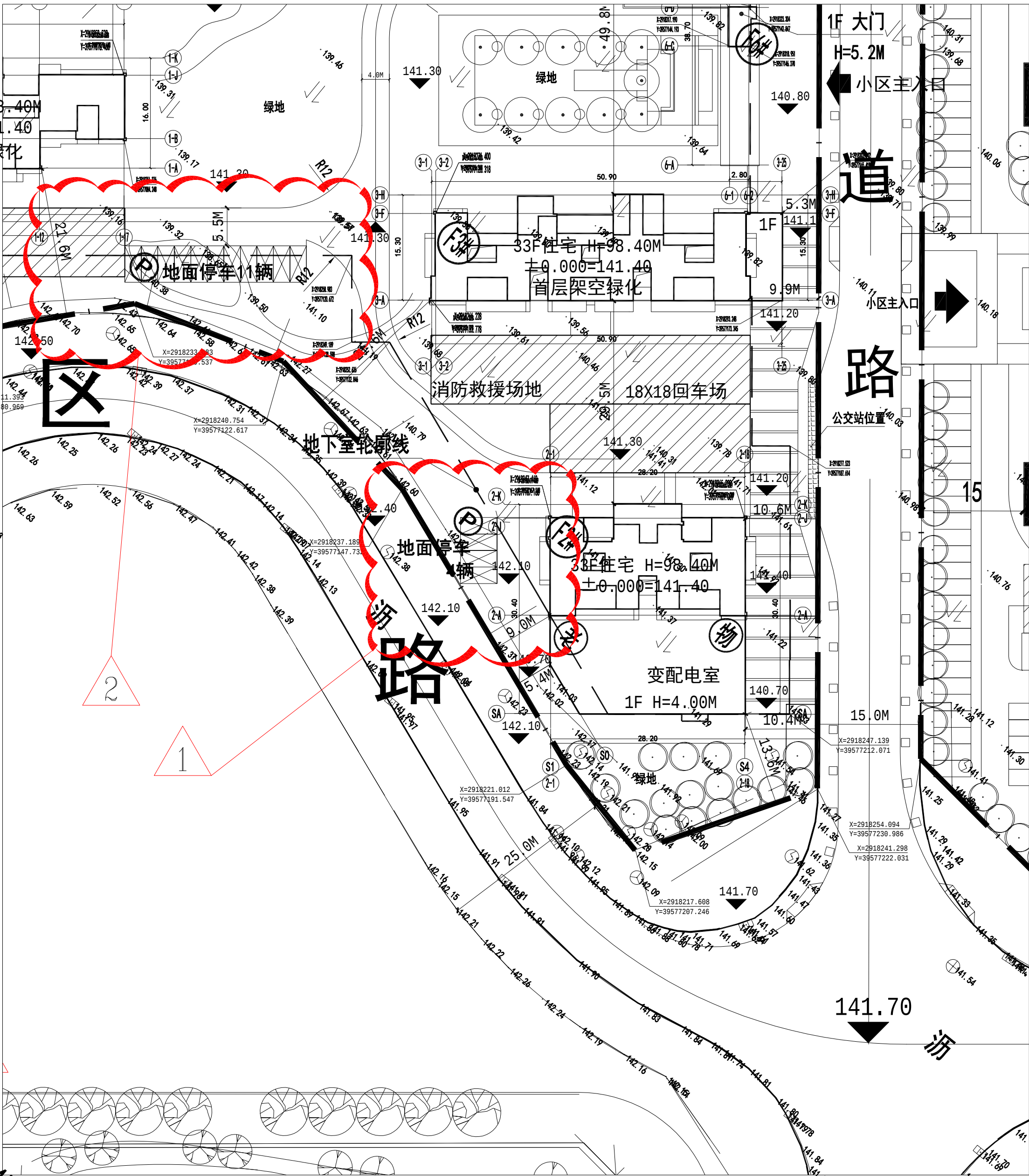
总平面局部平面图 1:500 (原审批图)
