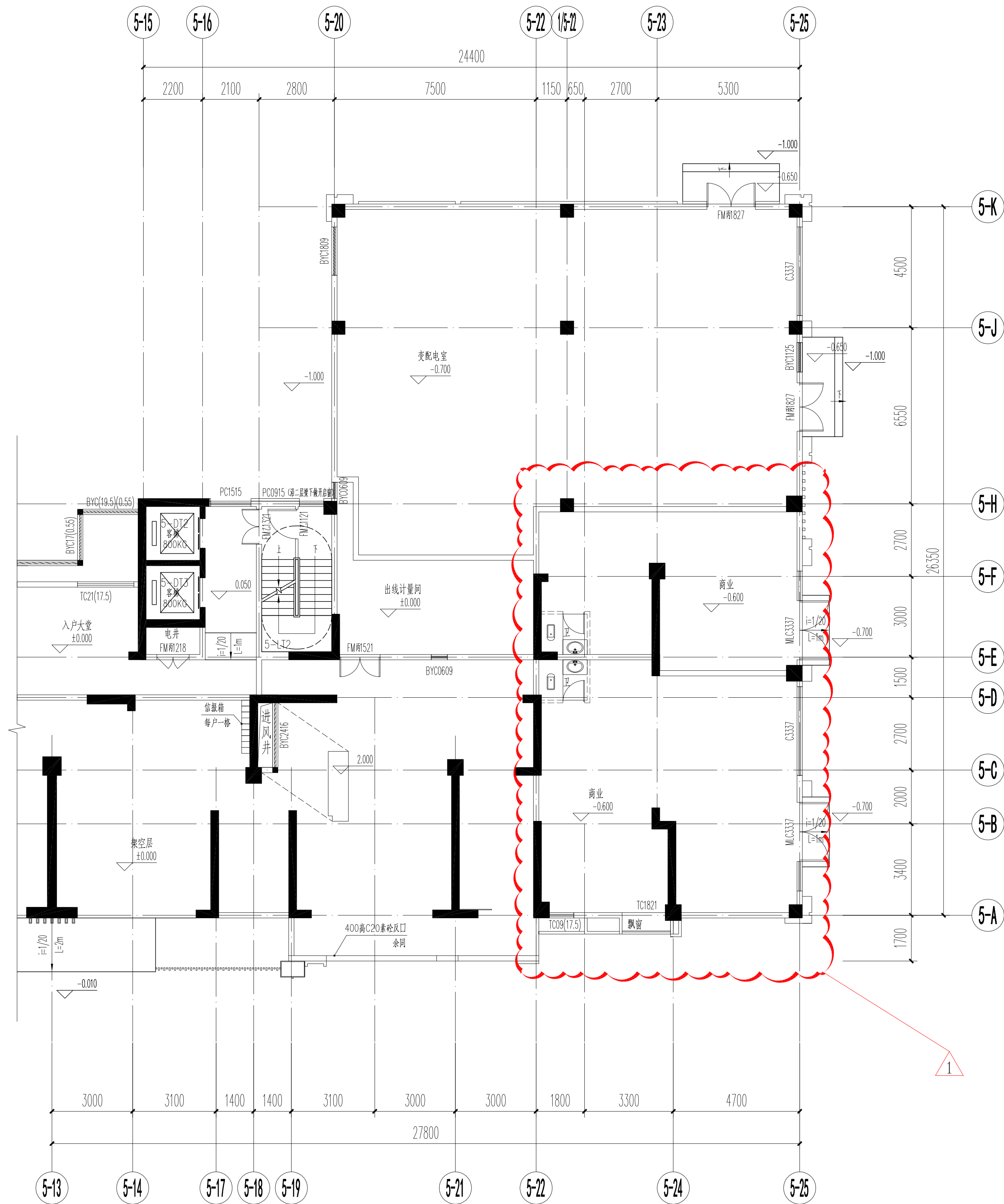
F5#楼一层局部平面图 1:100 (原审批图)
