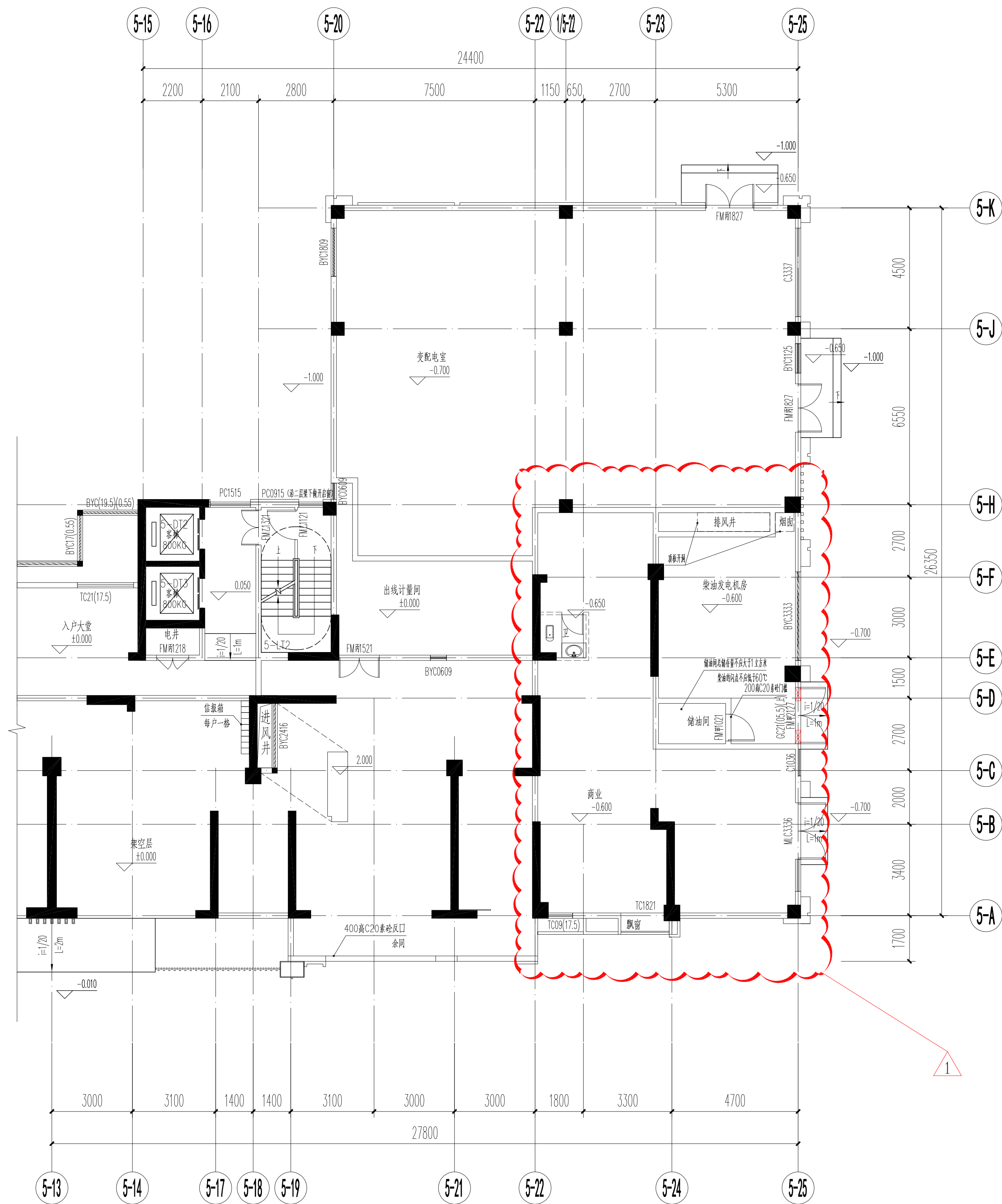
F5#楼一层局部平面图 1:100 (拟变更图)
