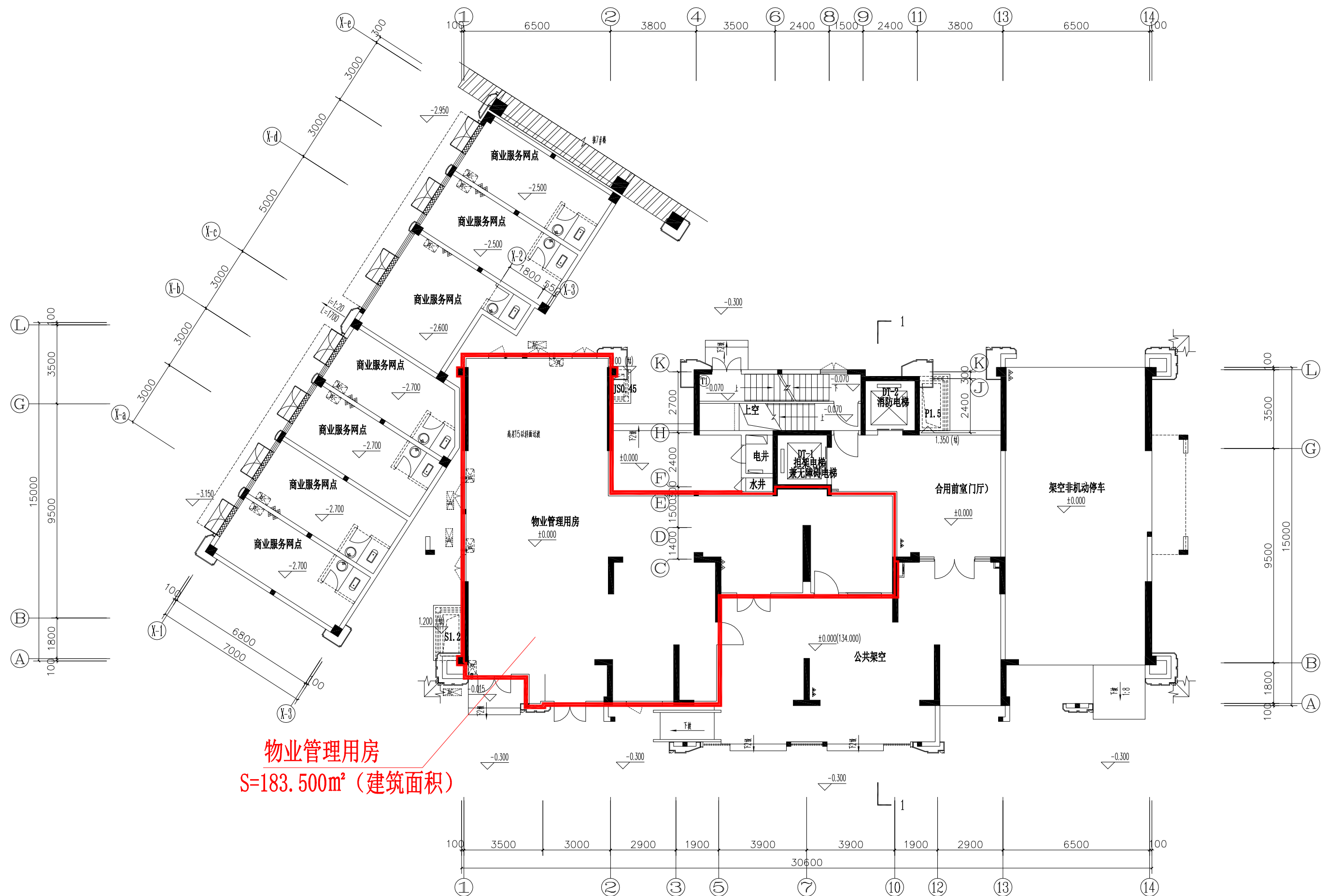
6#楼一层平面图
