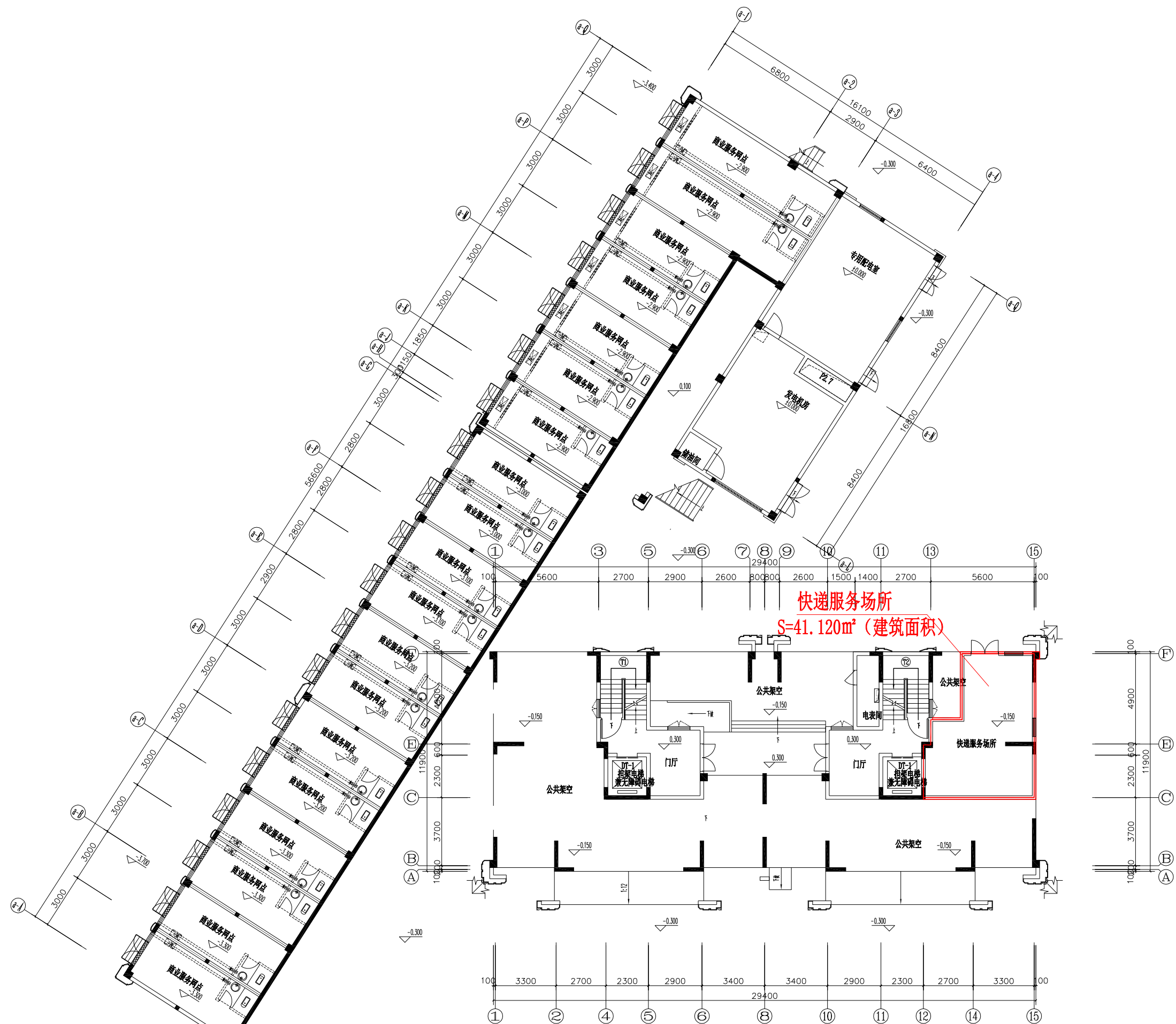
5#D3#楼一层平面图
